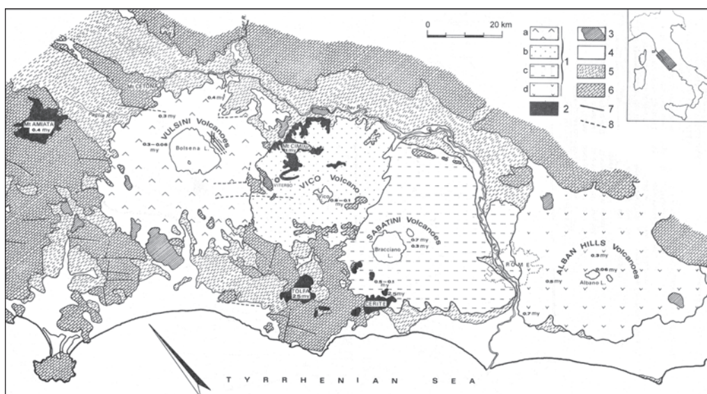
Fig. 1 - Schema geologico del dominio vulcanico laziale. 1) Vulcaniti alcalino potassiche (Quaternario) (a - Distretto Vulcanico dei Monti Vulsini; b - Distretto Vulcanico dei Monti Vicani; c - Distretto Vulcanico dei Monti Sabatini; d - Distretto Vulcanico dei Colli Albani); 2) Vulcaniti acide (Pliocene-Pleistocene); 3) Travertino; 4) Sedimenti continentali e costieri (Quaternario); 5) Sedimenti argillosi e sabbiosi (Miocene superiore-Pliocene-Pleistocene inferiore); 6) Successioni prevalentemente sedimentarie (Carbonifero-Miocene inferiore); 7) Faglie; 8) Faglie sepolte (Locardi et al., 1976).
